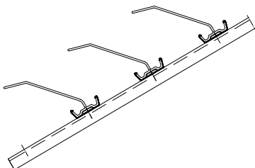
Widerstandsfähig gegen Feuer von außen, geprüft für Lamellenabstand 60 mm nach DIN V ENV 1187 (ersetzt DIN 4102-7) Prüfberichts-Nr. 233336414
